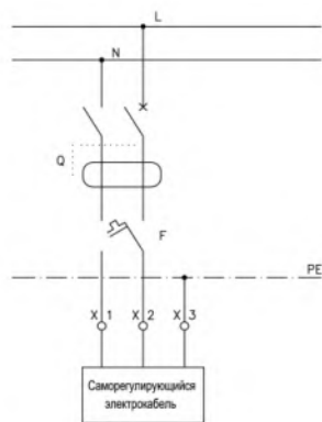
Рис. 2. Схема подключения электрообогрева кровельной воронки HL64.1H к электрической сети.
